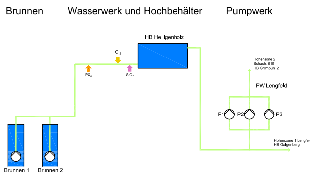
Verfahrensschema WW-E
