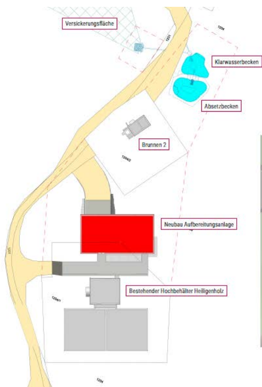
Bauplanung der Trinkwasseraufbereitungsanlage zur Trübstoffentfernung
