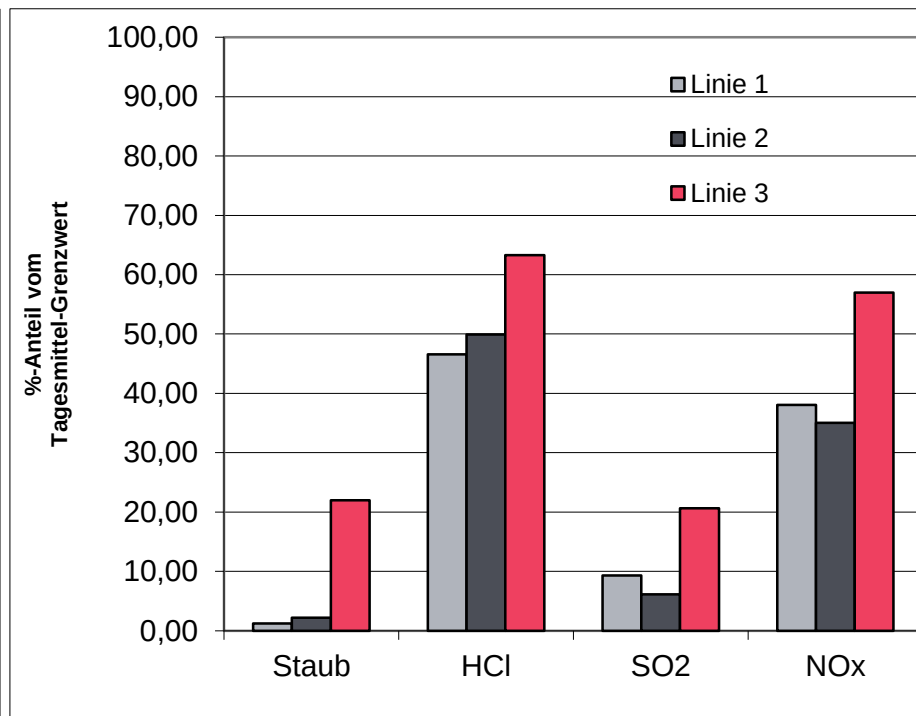
Grenzwerte der Tagesmittelwerte nach der 17. BImSchV
